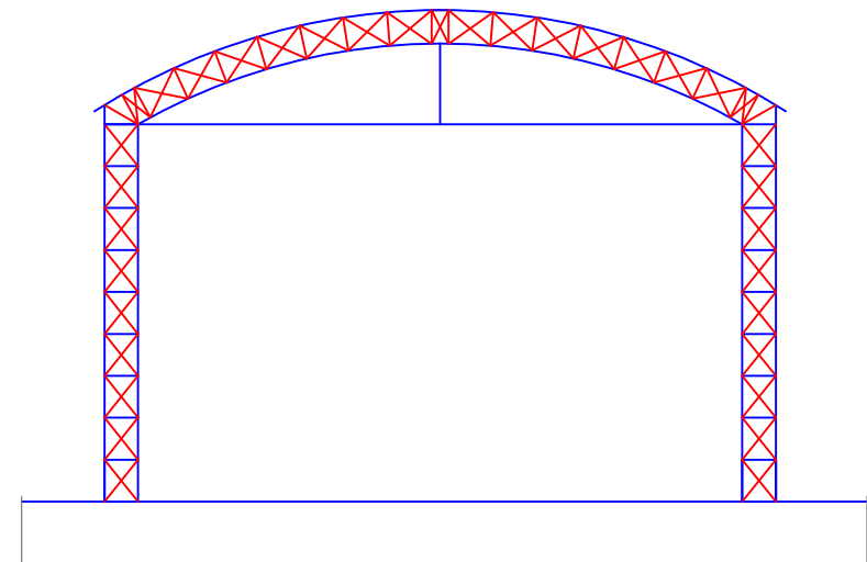
CORTE TRANSVERSAL Sem Escala
