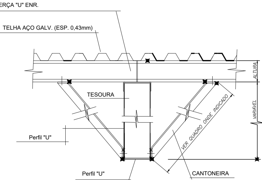
DETALHE MÃO FRANCESA S/ ESCALA
