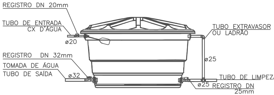
DETALHE LIGAÇÃO CAIXA D'ÁGUA SEM ESC.
