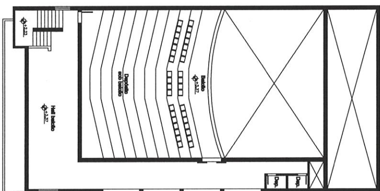
0 1 2 3 4 m PLANTA BAIXA - 1º PAV. Escala: 1/100
