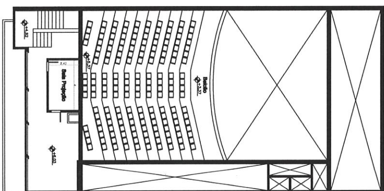
0 1 2 3 4 m PLANTA BAIXA - 2º PAV. Escala: 1/100
