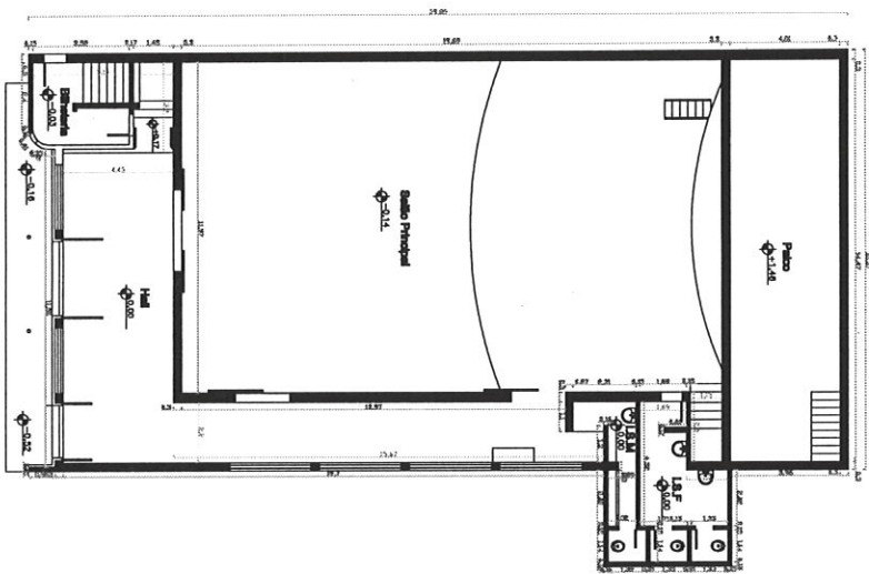
0 1 2 3 4 m PLANTA BAIXA - PAV. TÉRREO Escala: 1/100
