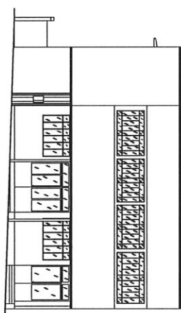
0 1 2 3 4 m FACHADA Escala: 1/100
