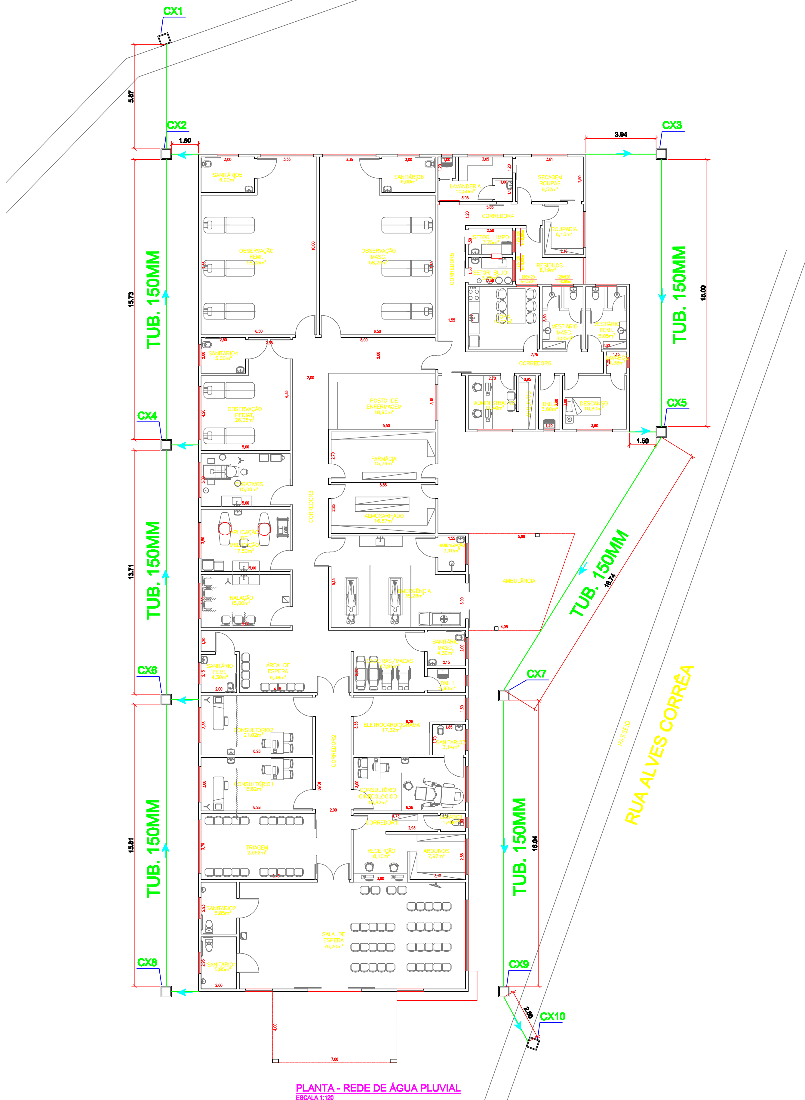
PLANTA - REDE DE ÁGUA PLUVIAL ESCALA 1:120
